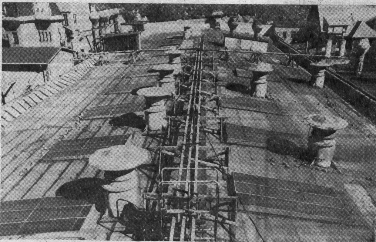
Die Erneuerung des Formereihallendaches unseres Betriebes erweist sich als eine komplizierte Aufgabe mit hohen Anforderungen. Ein überbetriebliches Neuereraktiv arbeitet an einer völlig neuen Demontagevariante des alten Daches.
