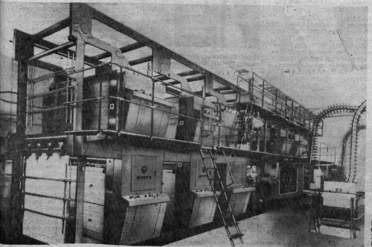
Der „Hyperset 1700“ wurde in den 60er Jahren der Übergang vom Hochdruck zum Offsetdruck in der Zeitungsherstellung vollzogen. Seit dem 8. Januar 1968 erscheint das „Neue Deutschland“ im Offsetdruck.
