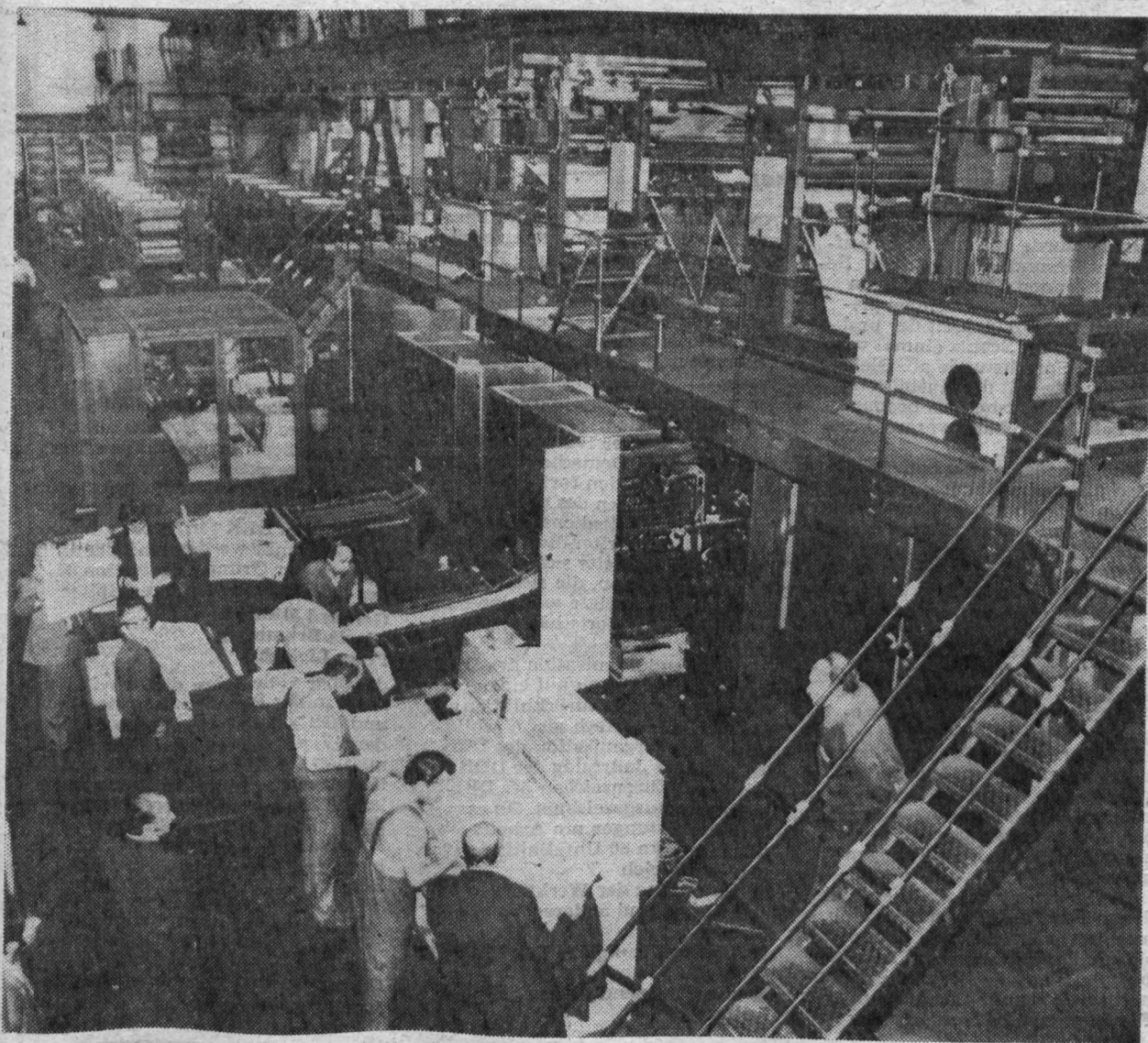
Die Abnahme der ROM Typ Noraset RO 130/70 für die Druckerei Szikra Budapest am 8. September in unserem Betrieb. Unser Bild zeigt die Hochleistungsmaschine in Paterreausführung für 32 Seiten (Standardformat). Der Technische Direktor der Druckerei, Genosse Josef Sandor, wertete mit Druckinstrukteur Dipl. Ing. Peter Elschner das Druckergebnis bzw. Falzprodukt aus. Dieses Ergebnis wurde auch dem ASMW zur Prüfung auf das Gütezeichen „Q“ vorgestellt. Wir hoffen auf Erteilung dieser Qualifikation.
