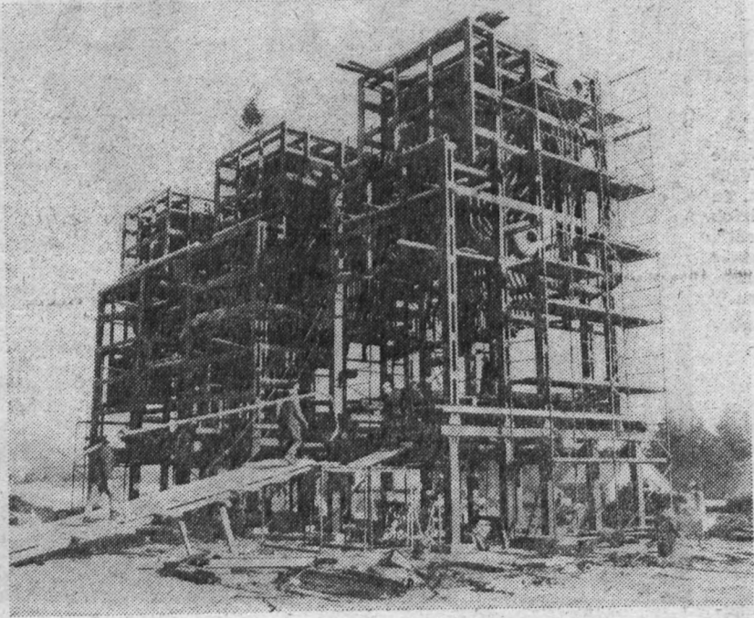
Unsere Archivfotos auf dieser Seite vermitteln einen kleinen Einblick in die umfassende komplexe Rationalisierung und Erweiterung der Plamag. Dieses Foto entstand am 10. Dezember 1968 und zeigt den Bau des Heizhauses.
