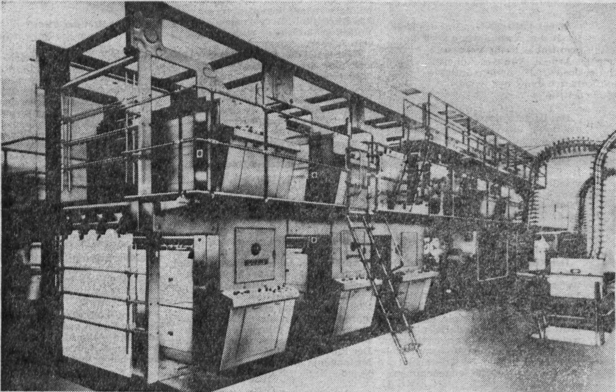
Das ist die Plamag-Zeitungsrollen-Offsetmaschine Hyperset 1700, mit deren Produktion 1963 begonnen wurde.
