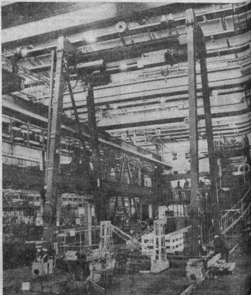
Mit diesem Vollportalkran konnte die Montagetechnologie in unserem Betrieb weiter qualifiziert werden. Der damit ermöglichte Komplettversand doppelbreiter RO-Maschinen führte zur bedeutenden Einsparung von Verpackungsmaterial und Transportraum.
