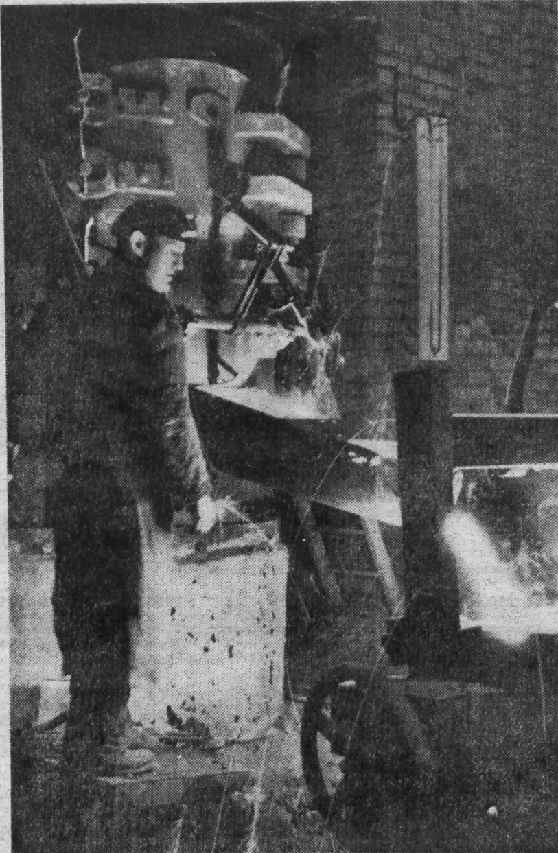
Historische Fotos aus der Entwicklung unseres Betriebes: Im Dezember 1947 wurde der Abstich des ersten Eisens von Kollegen Ernst Spitzbarth vorgenommen. (Von diesem Eisen wurde vor dem Vergießen eine Keilprobe gegossen.)
