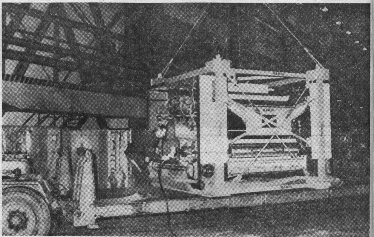
Durch den Komplettversand die Montage weiter zu rationalisieren, ist eine der vielfältigen Aufgaben, die im Wettbewerbsprogramm unseres Betriebes für 1982 gestellt sind. So ist u. a. vorgesehen, erstmals eine Riga-Maschine im Komplettversand nach Vilnius in die Sowjetunion zu liefern. Unser Foto zeigt den Komplettversand eines Druckwerkes für eine Maschine in die VR Polen im vergangenen Jahr.
