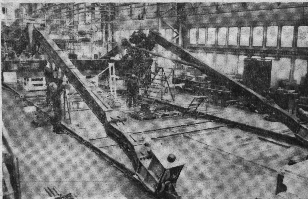
Unser Bild zeigt die Montage eines Vollportalkrans als Gemeinschaftsobjekt territorialer Rationalisierung mit dem VEB MLK Plauen. Dieser Kran ist eine Voraussetzung für die weitere Qualifizierung der Montagetechnologie. Das ermöglicht in diesem Jahr den Komplettversand doppelbreiter RO-Maschinen in die Sowjetunion und nach Finnland. Damit wird eine Maßnahme aus dem Kampfprogramm der BPO für 1982 realisiert.
