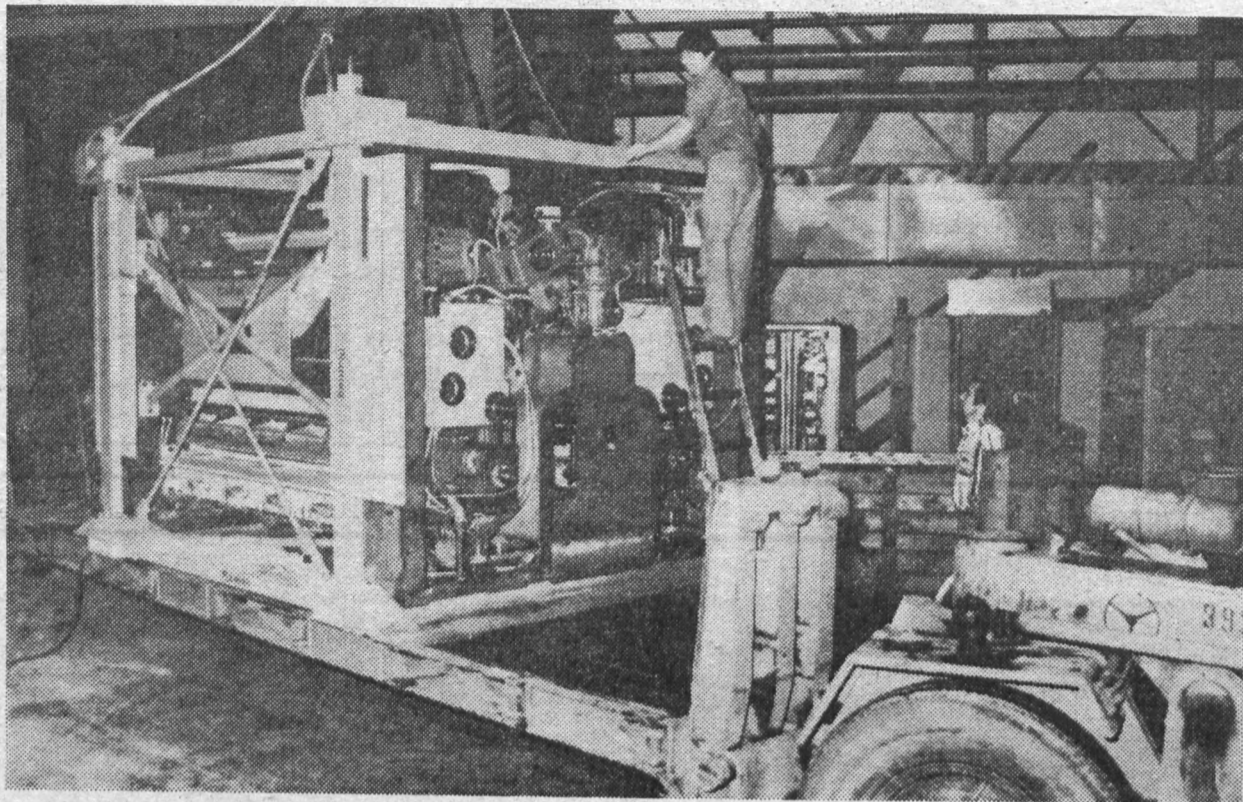
Unser Foto zeigt den Versand eines Druckwerkes für eine Maschine für die Volksrepublik Polen. Mit diesem Ende August praktizierten Komplettversand können Druckmaschinenaggregate bis zu 22 t ohne Demontage transportiert werden.
