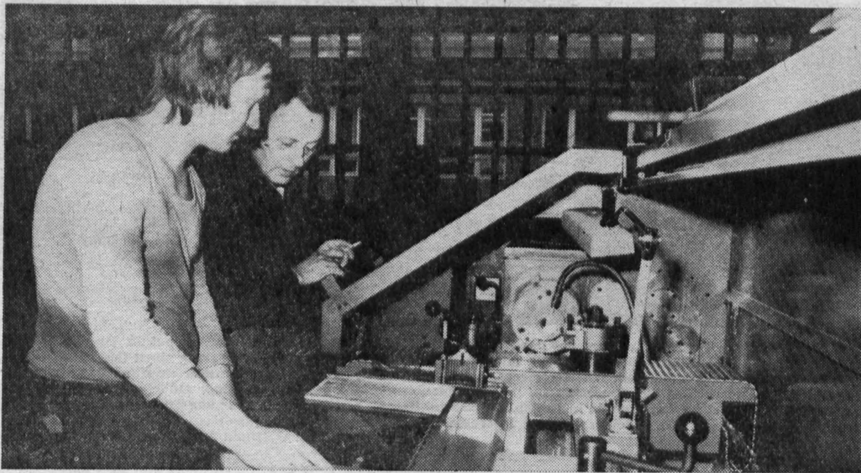
Obiges Foto zeigt eine der zwei CNC-Drehmaschinen (rechnergesteuerte Drehmaschinen), die seit einigen Tagen in der Revolverdreherei unseres Werkes zum Einsatz gekommen sind. Genauer gesagt befinden sich beide Maschinen im Erprobungsstadium. Erwartet wird von dieser modernen Technik eine Steigerung der Arbeitsproduktivität sowie eine Arbeitserleichterung für den Bediener. Hier weist der ungarische Monteur Bliznik Genossen Wenda in die Bedienung der Maschine ein.
