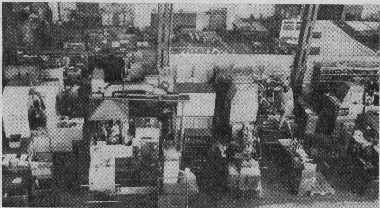
Blick in die Verzahnteilefertigung im FB 2. Das Charakteristische dieses Fertigungsabschnittes ist, daß dort in Mehrmaschinenbedienung gearbeitet wird. Foto: K.-H. Dreßel
