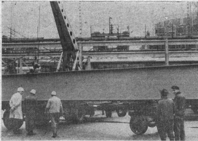
Dieser Riese, ein Kranbahnträger von 18 m Länge, der im Hauptwerk in der Hammerstraße gefertigt wurde, verläßt die Werkstatt und wird zum WT V in die Auenstraße gebracht.
