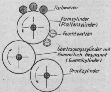
Abb. 1. Offsetdruck. Druckvorgang
